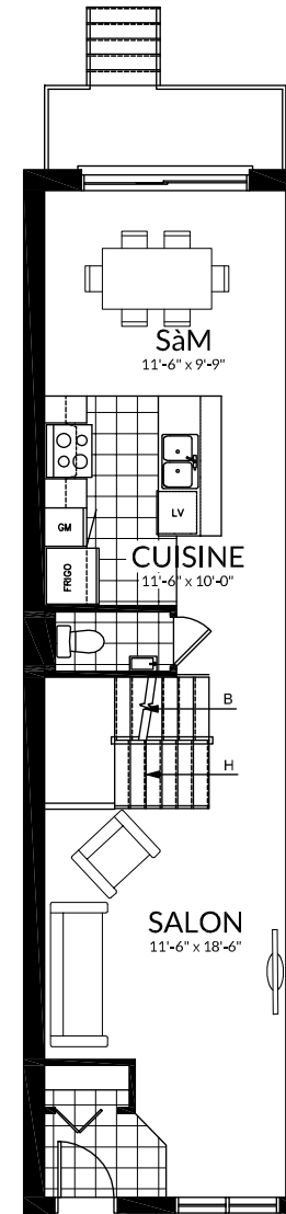
REZ-DE CHAUSÉE
