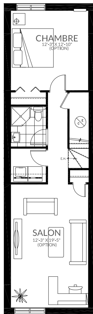
SOUS-SOL
