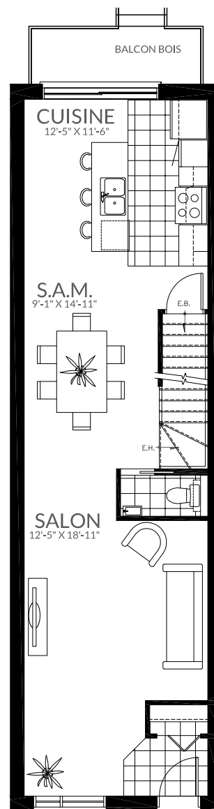
REZ-DE CHAUSÉE
