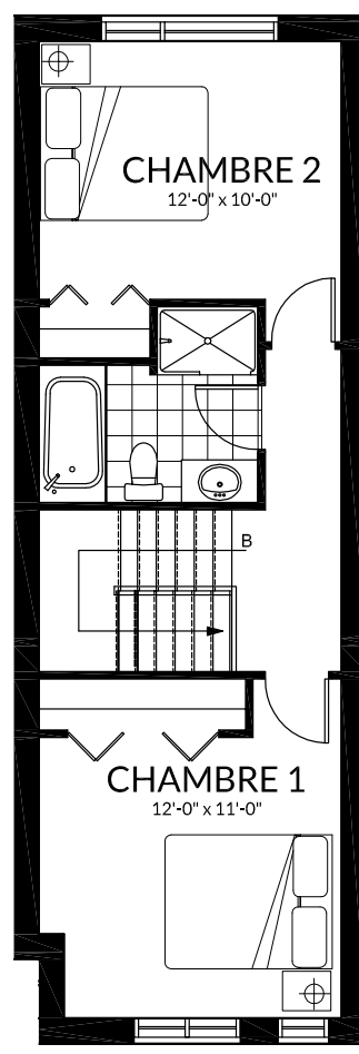
ÉTAGE
