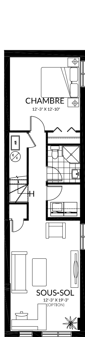
SOUS-SOL
