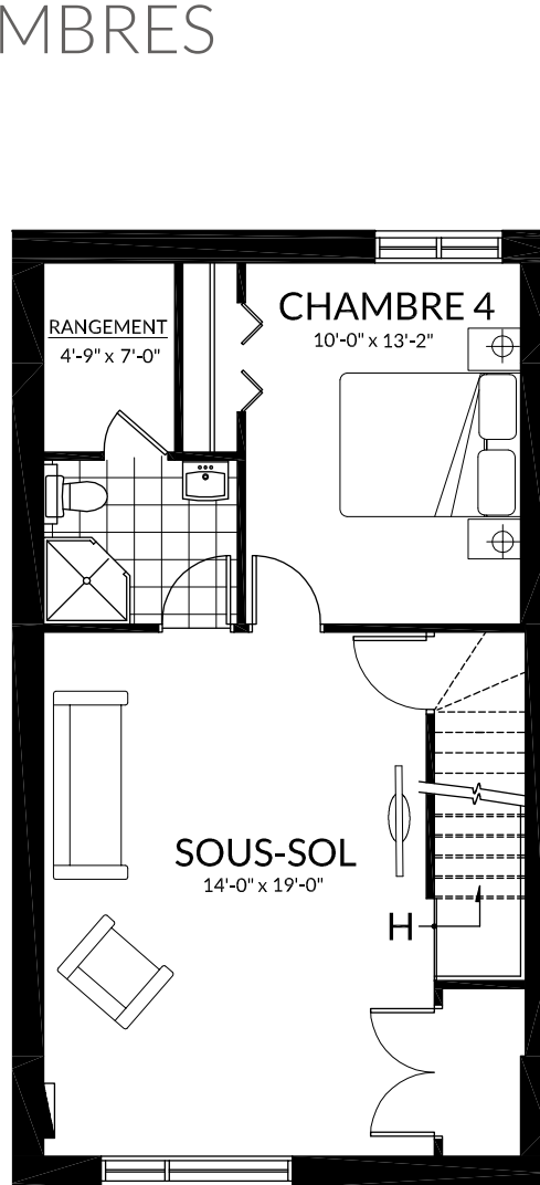
SOUS-SOL
