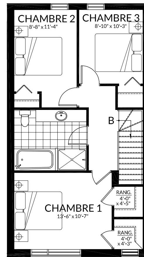
ÉTAGE
