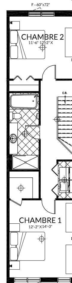
ÉTAGE
