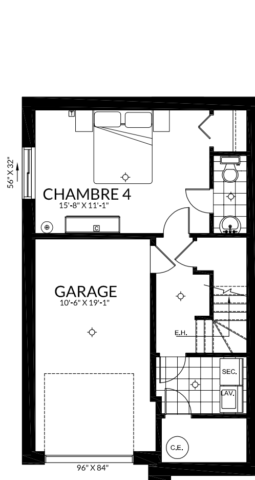
SOUS-SOL FINITION EN OPTION
