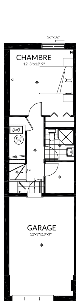
SOUS-SOL (Finition en option)
