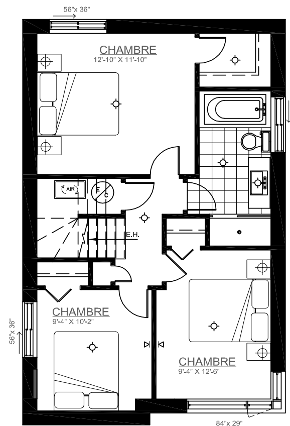
SOUS-SOL
