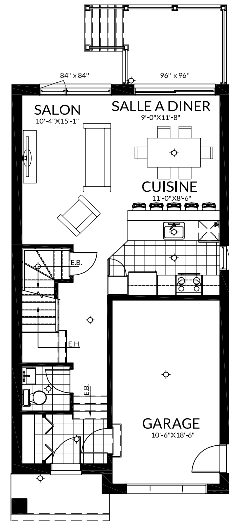
REZ-DE CHAUSÉE
