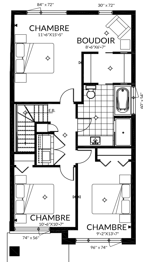
ÉTAGE
