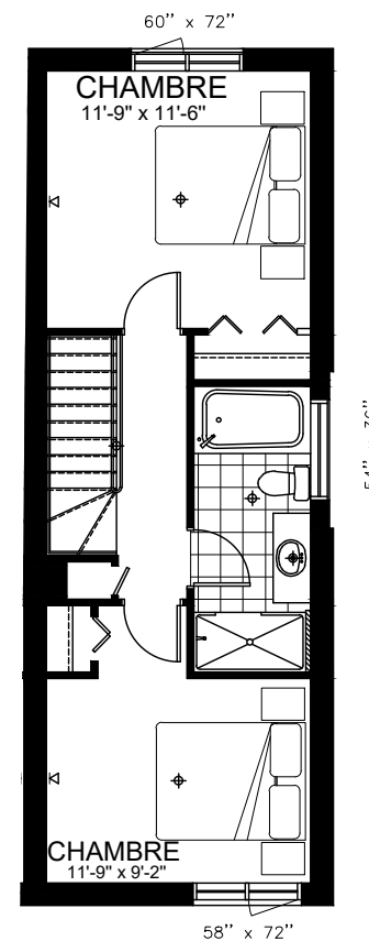
ÉTAGE
