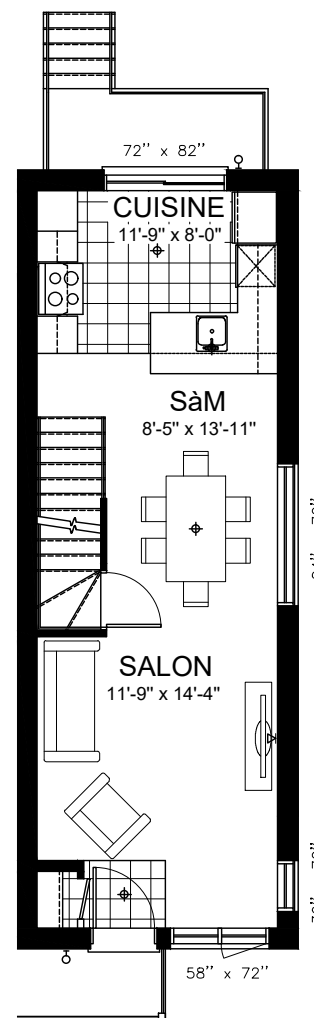
REZ-DE CHAUSÉE
