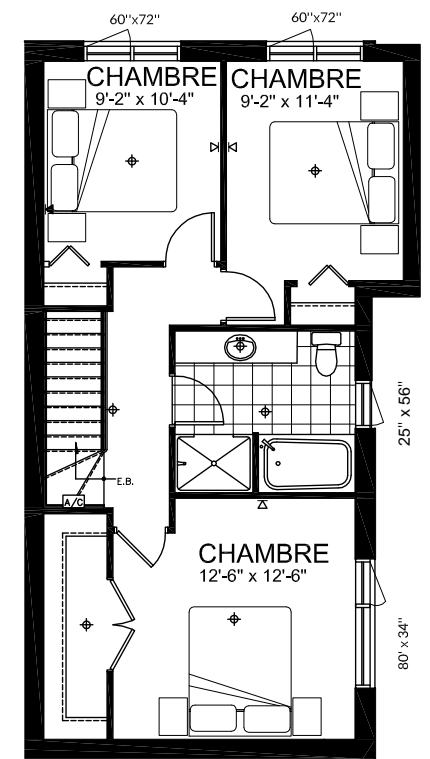
ÉTAGE
