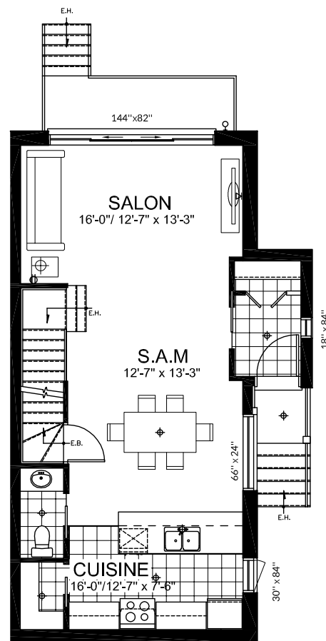
REZ-DE CHAUSÉE
