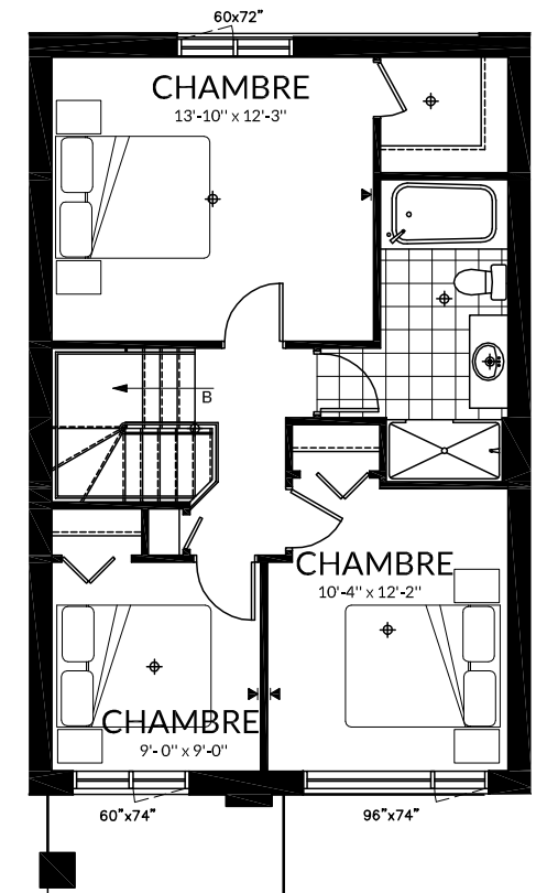
ÉTAGE
